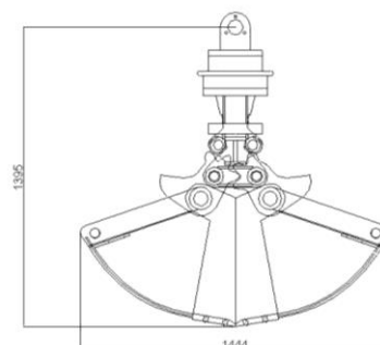
Bahngreifer 280 mm
